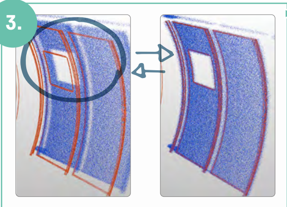
Automatisches 3D-Matching mit CAD-Modell.
