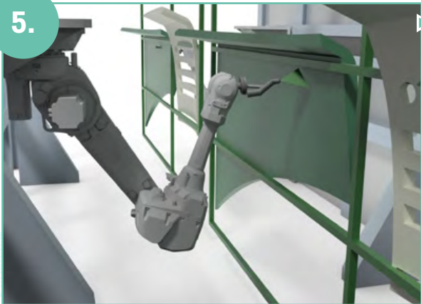
Übermittlung realer Werkstückkoordination an Robotersteuerung.
