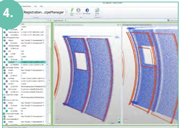
Berechnung der Lagekorrektur im Bauteil- oder Trägerkoordinatensystem.
