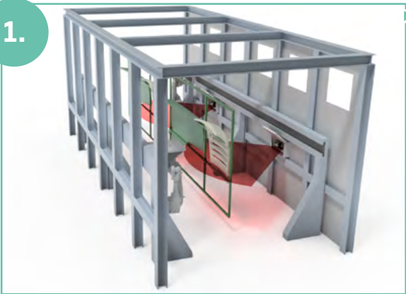
Bauteilscan vor oder innerhalb der Lackierkabine.
